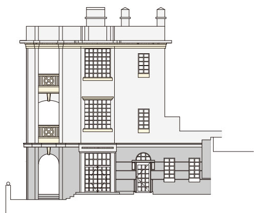
NORTH WEST ELEVATION 西北立面圖
